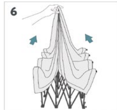
6 Commencer par resserrer la structure à moitié Répartir le visuel de façon uniforme sur la structure. Prendre le visuel au niveau des noeuds et le rassembler en un point. Close the frame halfway. Separate the graphic uniformly on the structure, then take the graphic and pull it up to a point.
